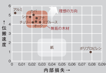
スピーカー素材の物性値(伝搬速度 対 内部損失)
