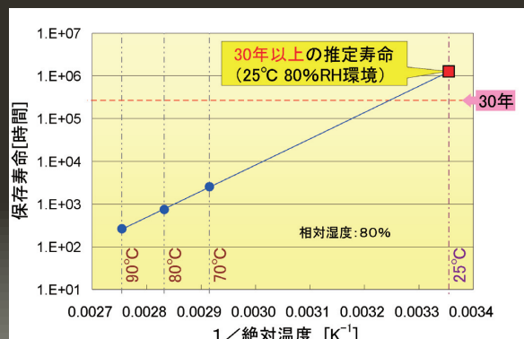
BD-R50GB アレニウス法による寿命推定結果(MTTF)
